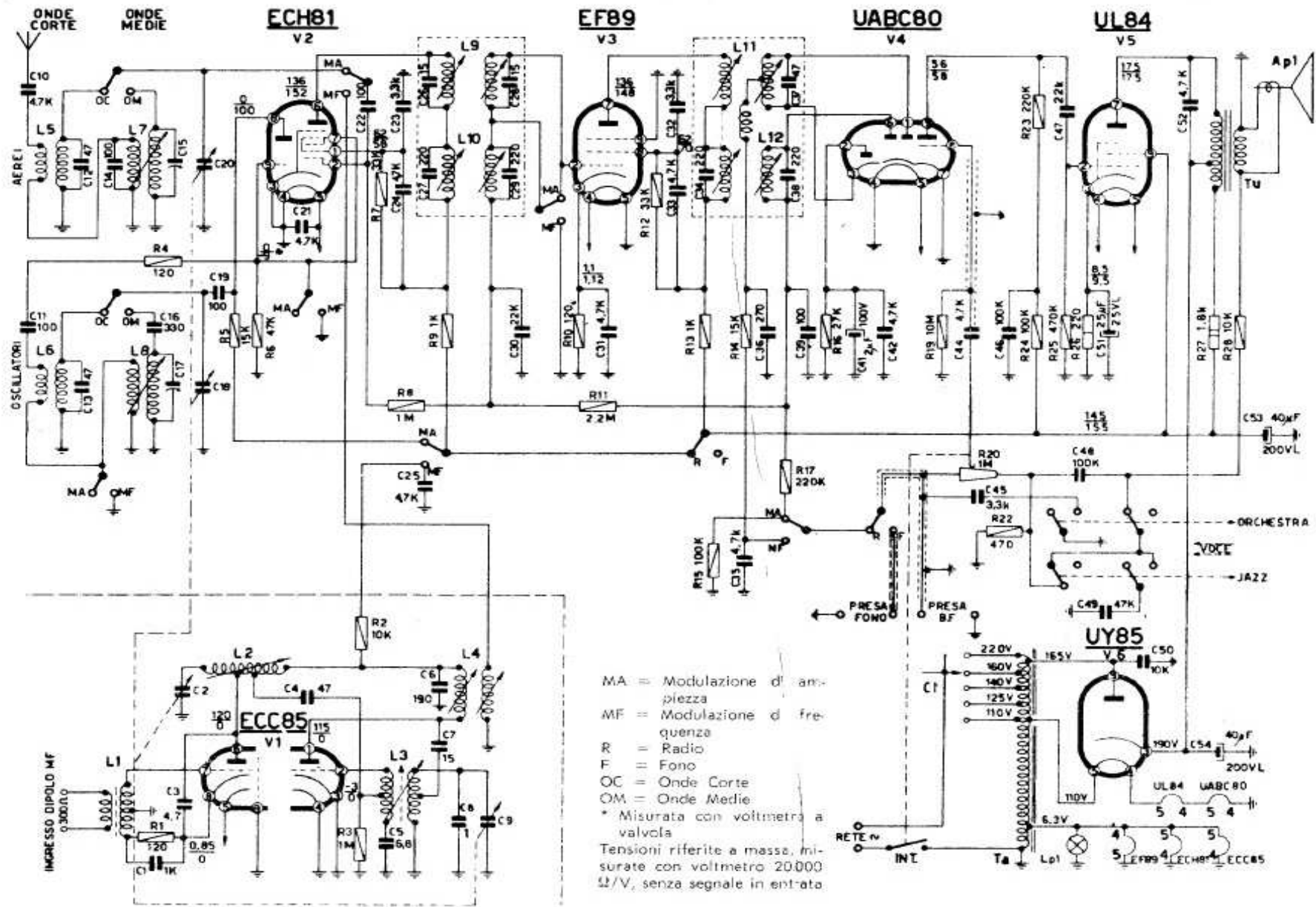
RADIORICEVITORI ALLOCCHIO BACCHINI Mod. 450 - 1070 - 1072
